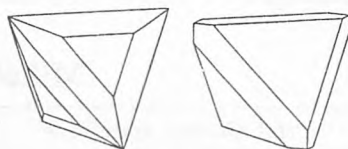
Kryształy tetraedrytu
