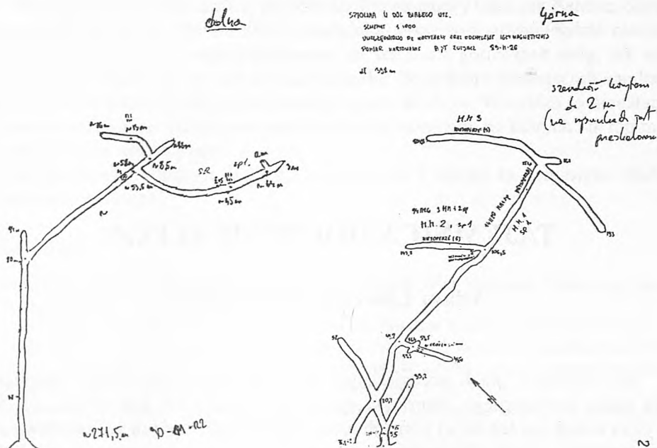
Pomiary i rysunki sztolni wykonał pracownik Tatrzańskiego Parku Narodowego, Tomasz Zwijacz-Kozica w roku 1997
