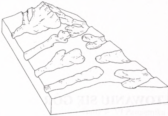
Schemat erozji wstecznej w masywie górskim prowadzącej do powstania ostrej grani i szczytów (wg Blooma)
