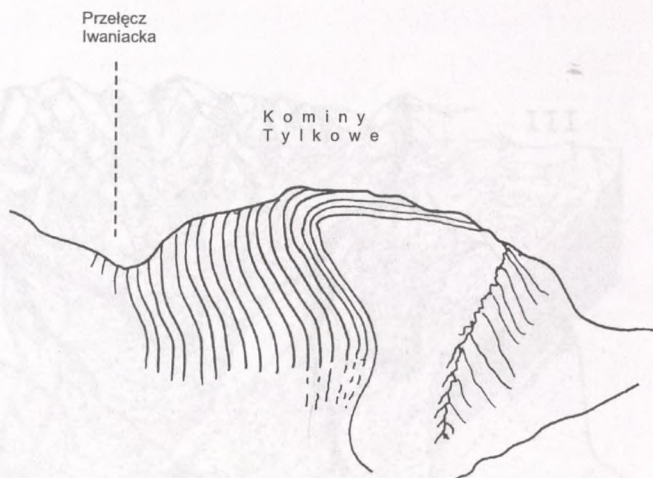
Zawinięcie warstw triasu na szczycie Kominów Tylkowych tworzące powierzchnię strukturalną
