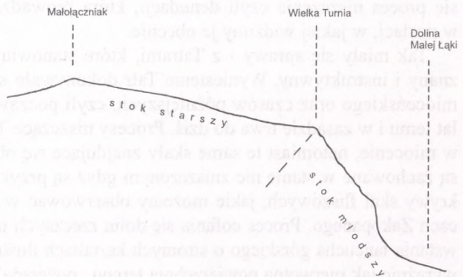
Zarys zbocza Małolączniaka ilustrujący względny wiek poszczególnych części zbocza
