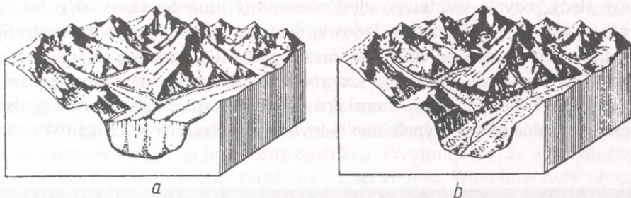
Dolina zlodowacona a – wypełniona lodowcem, b – po stopieniu lodu (wg Książkiewicza)
