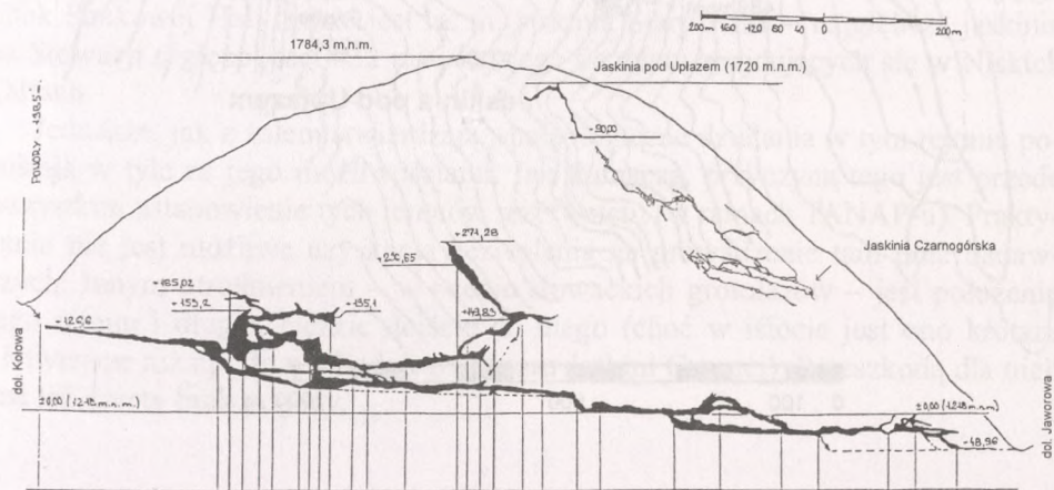
Przekrój masywu Czarnogórkskiej Czuby (1784 m n.p.m.) z Jaskinią Jaworzynki. Wg „Spravodaj Slovenskej Speleologickej Spoločnosti” 1996, nr 2, s. 8, uzupełniony o orientacyjny przekrój Jaskini Czarnogórkskiej i Jaskini pod Czarnogórkškim Uplazem
